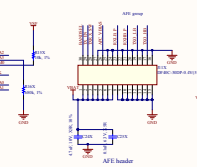
AFE header
